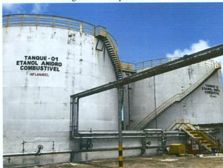
Figura 1 – Tanques Verticais
